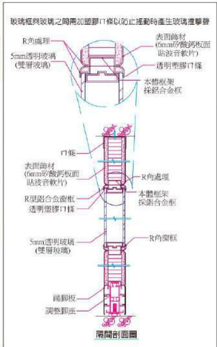
塊狀 R 系列矽酸鈣板高隔 (符合耐燃一級·鋁合金表面採陽極處理)
